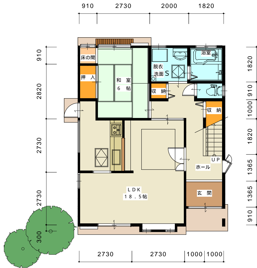
1階平面図 1/100
