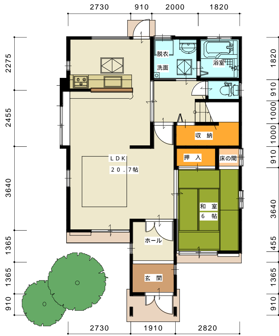
1階平面図 1/100
