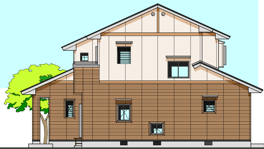
立面図 1/100
